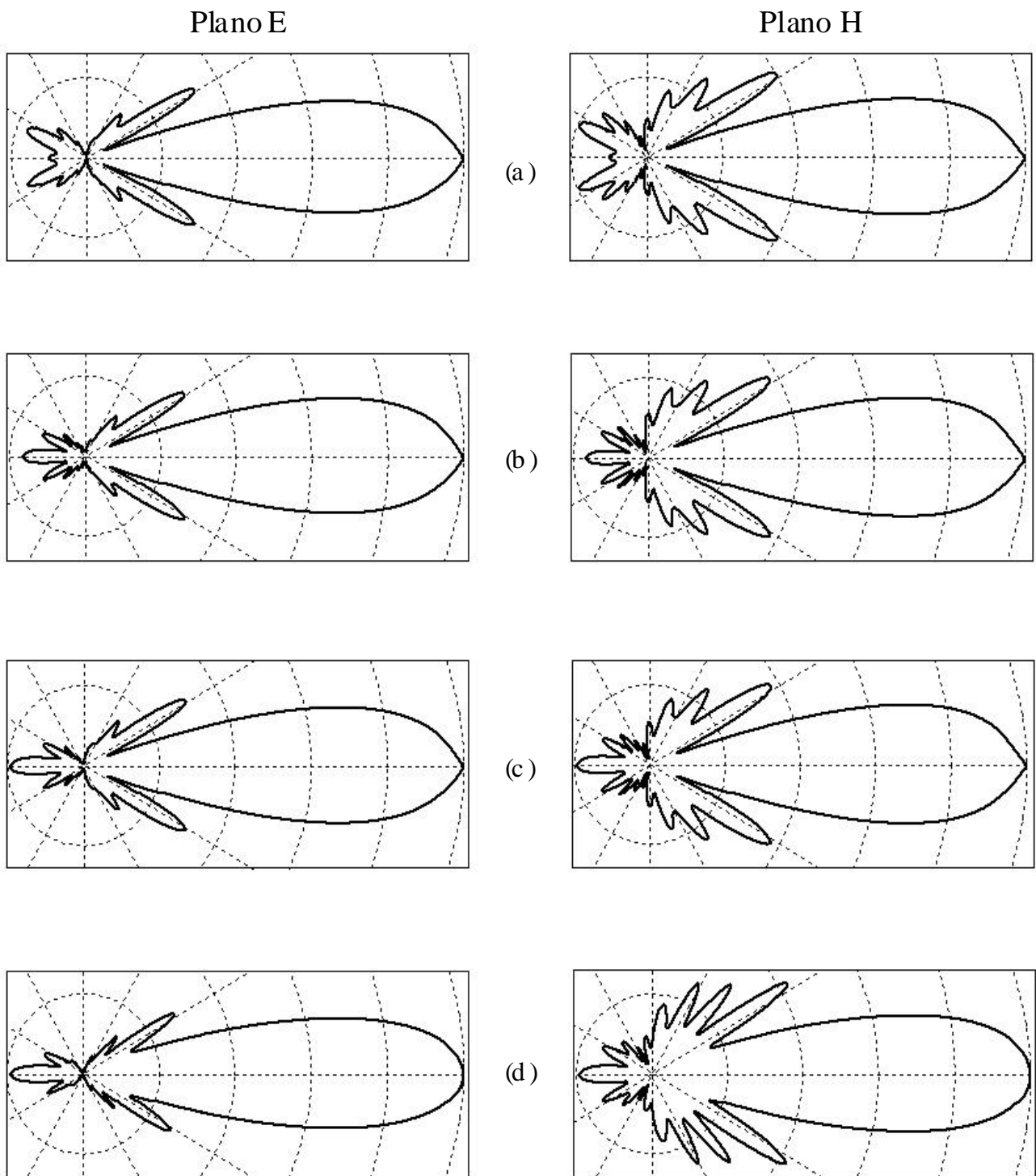
Figura 11. Patrones de radiación normalizados de campo eléctrico para arreglos Yagi resonantes con 15 elementos, alimentados con: a) Un dipolo recto, b) Un dipolo doblado coplanar alimentado en su brazo izquierdo, c) Un dipolo doblado coplanar alimentado en su brazo derecho; y d) Un dipolo doblado transversal
