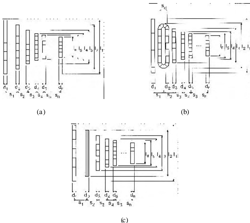
Figura 3. Variables de longitud, diámetro y separación utilizadas en el análisis por el método de momentos. a) Alimentación con dipolo recto sencillo ( 2^{\circ} elemento), b) Alimentación con dipolo doblado coplanar; y c) Alimentación con dipolo doblado transversal. Todos los elementos se muestran segmentados de acuerdo con los requerimientos del método de momentos, la segmentación utilizada para el dipolo doblado coplanar es la misma que en el dipolo transversal, solo que éste último se muestra en gris, debido a la dificultad de representarlo en forma segmentada (Ver Figura 2d)
