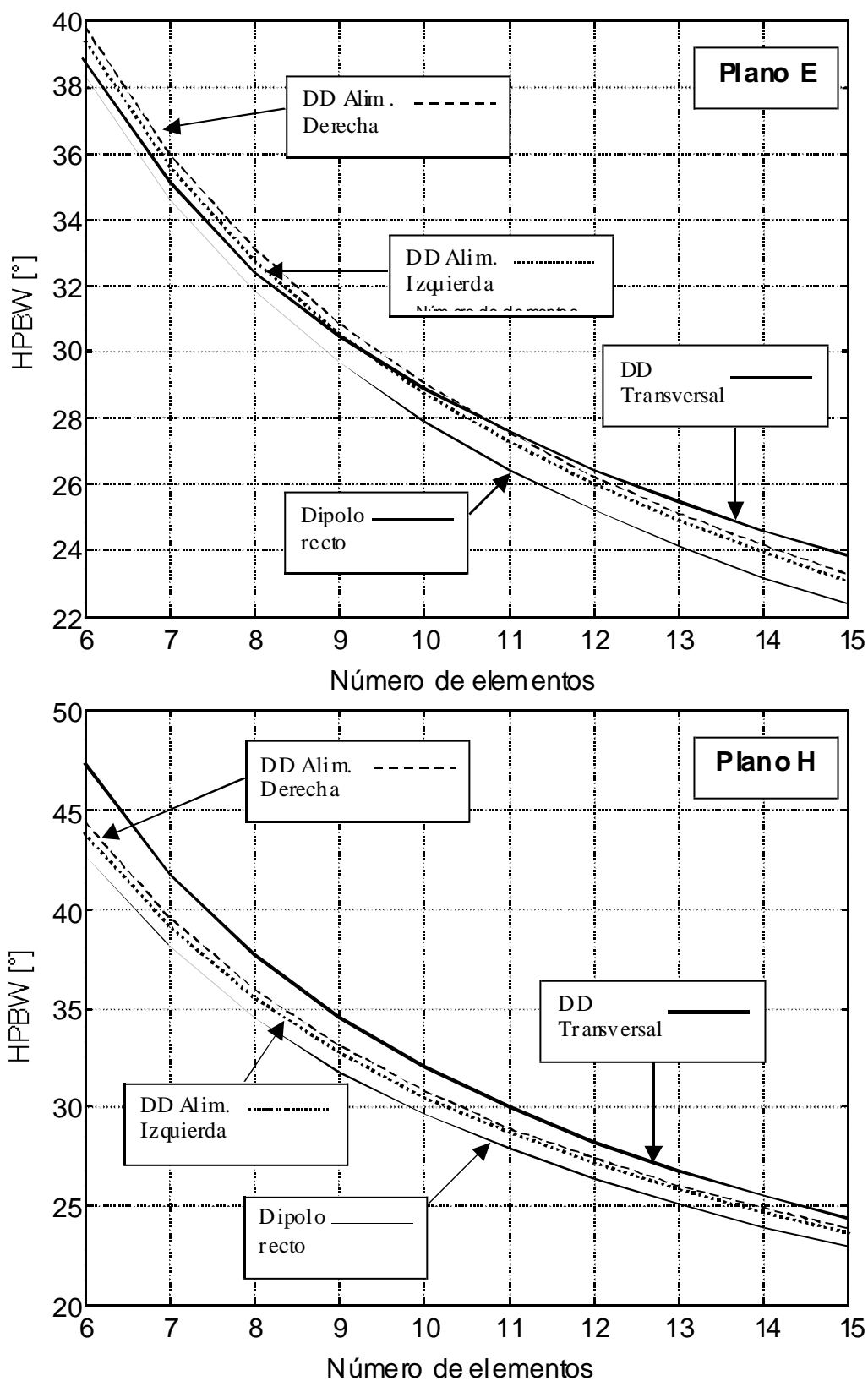
Figura 9. Ancho del haz de media potencia (HPBW por sus siglas en inglés) de los arreglos Yagi resonantes con las dimensiones presentadas en la tabla 1 s_d=0.083\lambda
