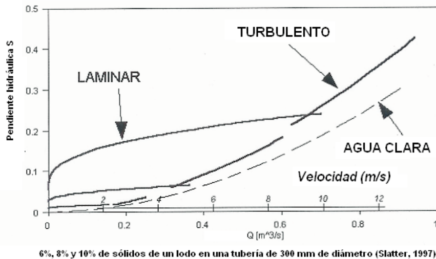
6%, 8% y 10% de sólidos de un lodo en una tubería de 300 mm de diámetro (Slatter, 1997)
