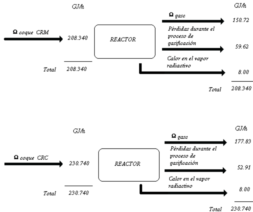
Figura 2. Balance térmico para el proceso de la gasificación del coque CRM y CRC
