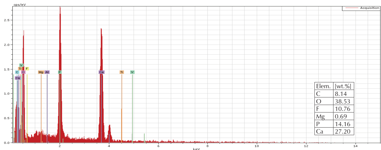
Figura 8. Espectro y análisis cuantitativos realizados en la partícula de hueso
