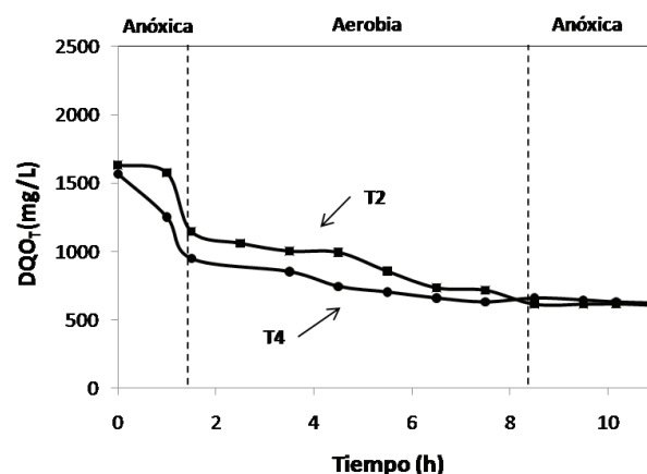
Figura 3. Evolución de la DQO_7 durante un ciclo de operación del SBR para los tratamientos T2 y T4
