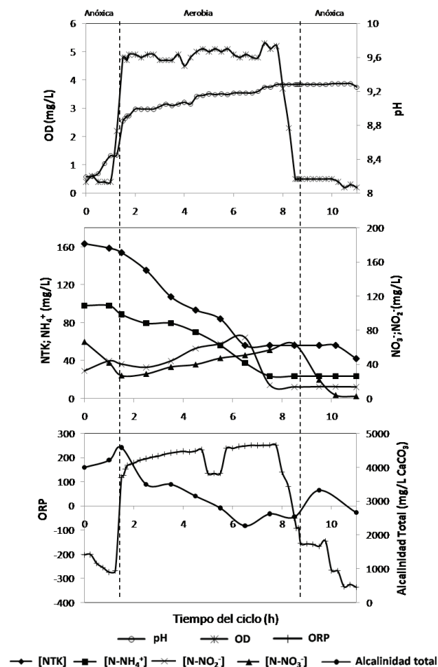
Figura 8. Perfil de las concentraciones de NTK, N-NH_4^+ , N-NO_3^- , N-NO_2^- , pH, OD, ORP y alcalinidad total durante un ciclo de 11 h durante el tratamiento T3 en el SBR
