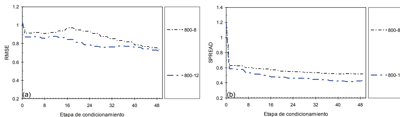
Figura 7. Evolución del error en la estimación del campo de referencia de log-permeabilidades en las diferentes etapas de condicionamiento utilizando 8 y 12 historias piezométricas con 800 realizaciones del campo aleatorio inicial de parámetros, a) evolución de la medida RMSE, b) evolución de la medida SPREAD
