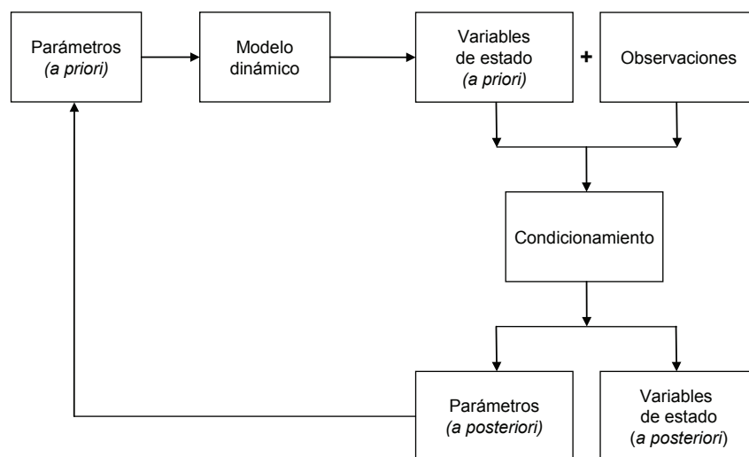
Figura 1. Diagrama conceptual del método EnKF
