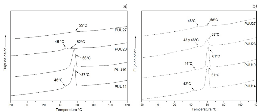
Figura 4. Termogramas de fusión de muestras de PUUs con diferentes porcentajes de SR: a) tratamiento de 0 días y b) de 140 días en PBS
