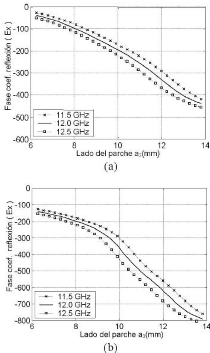
Figura 14. Fase del coeficiente de reflexión para la estructura de la Fig. 13, en función del lado de los parches. (a) 2 capas ( a_1 = 0.7a_2 ), (b) 3 capas ( a_1 = 0.7a_3 , a_2 = 0.9a_3 )
