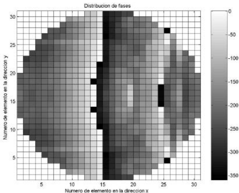
Figura 27. Distribución de fases para un haz lateral
