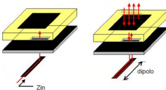
Figura 9. (a) Modelo de alimentación por línea microcinta. (b) Modelo de alimentación a través de una antena de tipo bocina (reflectarray)
