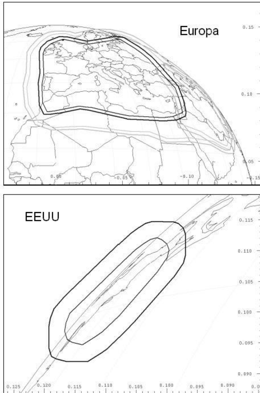
Figura 19. Coberturas para Europa y EEUU
