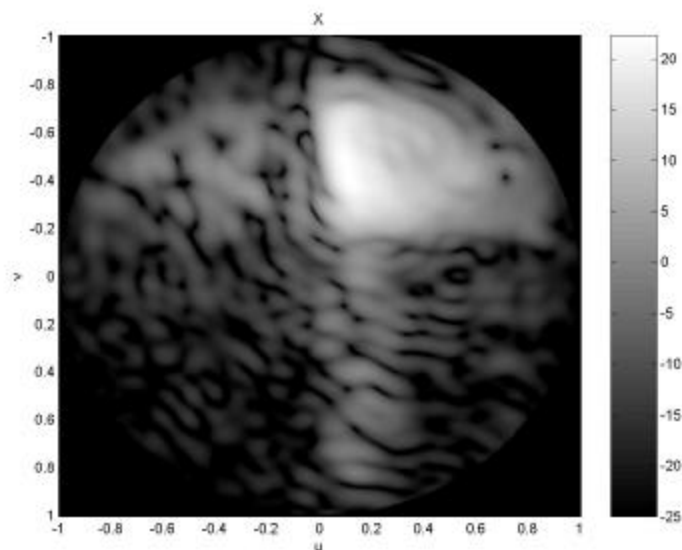
Figura 28. Patrón de radiación de un haz lateral
