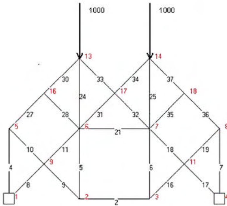
Figura 11. Armadura óptima, caso de estudio 3
