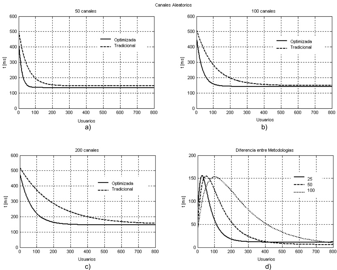
Figura 9. Resultados obtenidos al variar el número de usuarios para cambios a canales aleatorios: a) 50 canales, b) 100 canales, c) 200 canales, d) Diferencia entre ambas tecnologías
