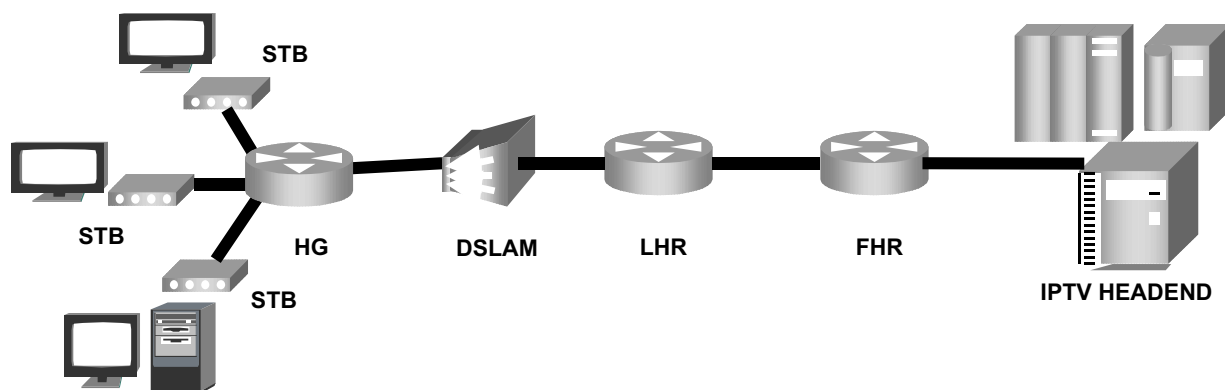
Figura 1. Arquitectura general del sistema IPTV
