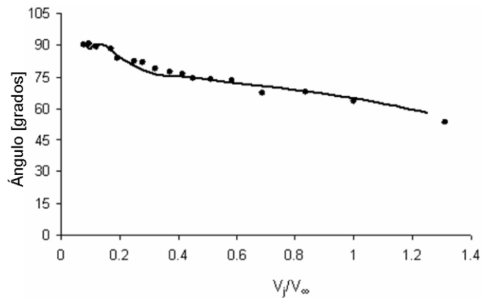
Figura 7. Ángulo de deflexión de llama con respecto a la relación de velocidades V_f/V_\infty . Predicciones (línea continua) y datos experimentales (puntos)
