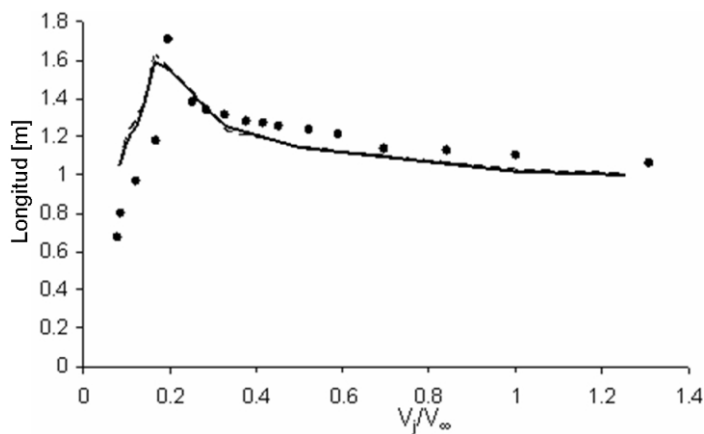
Figura 6. Longitud de llama con respecto a la relación de velocidades V_f/V_\infty . Predicciones (línea continua) y datos experimentales (puntos)
