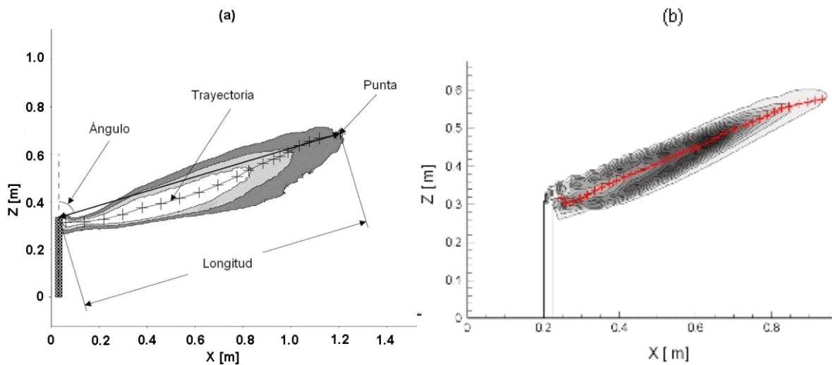
Figura 3. Perfil de la trayectoria media de la llama a una velocidad del flujo cruzado, V_f , de 2.0 m/s ( V_f/V = 0.5 ). a) Experimento (tomado de Majeski et al., 1999) y b) Modelo numérico
