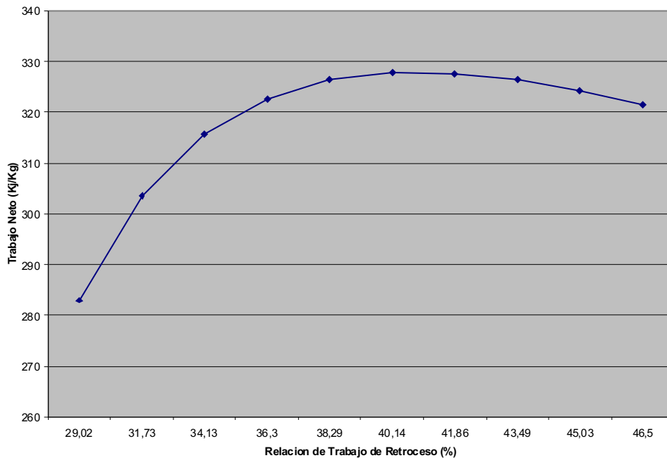
Figura 3. Variación del trabajo neto en kJ/kg versus la relación de trabajo de retroceso para el argón
