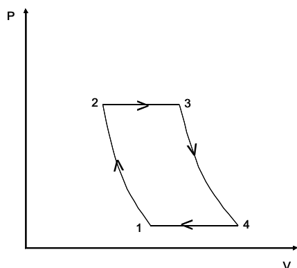
Figura 2. Diagrama P-V de un ciclo Brayton
