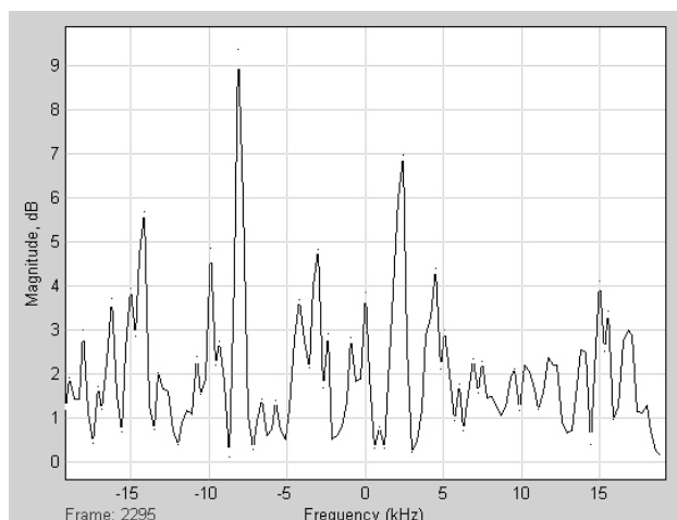
Figura 13. Espectro de la señal WCDMA en BB
