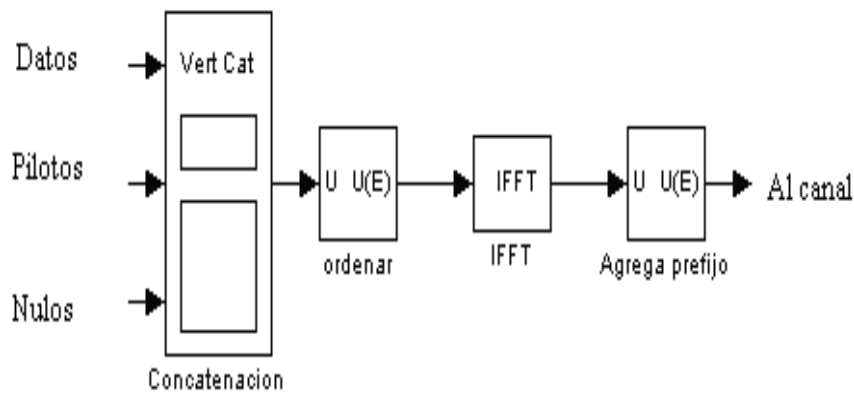
Figura 8. Bloque IFFT
