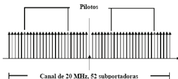
Figura 1. Distribución de subportadoras en OFDM
