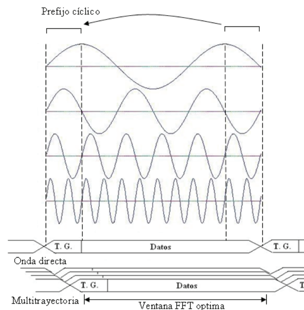
Figura 2. Extensión cíclica
