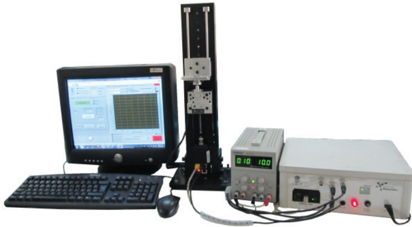
Figura 11. Equipo de microtensión MUA en funcionamiento
