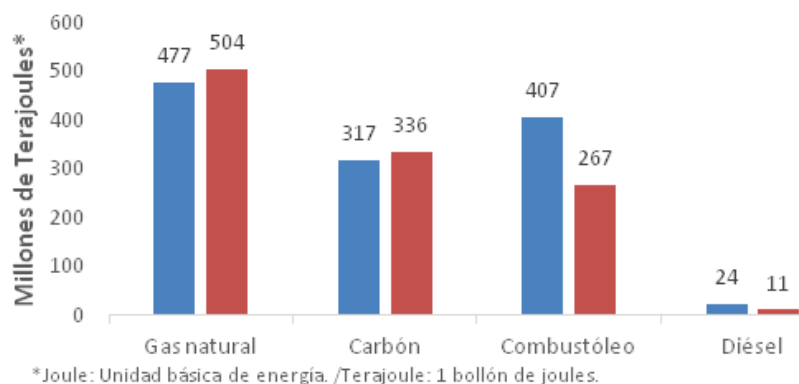
Figura 4. Consumo de combustibles fósiles para la producción de energía eléctrica en México (CFE, 2015)
